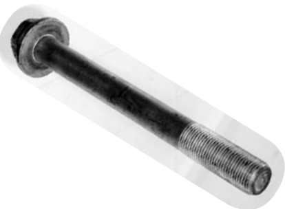
790.350 = PINO DO JUMELO DA MOLA DIANT. E TRAS. P/ TRAS. DELIVERY 11.160 APÓS 2018 (COMP. 147 MM) M18 X 1,5 N°. ORIG. ( )
